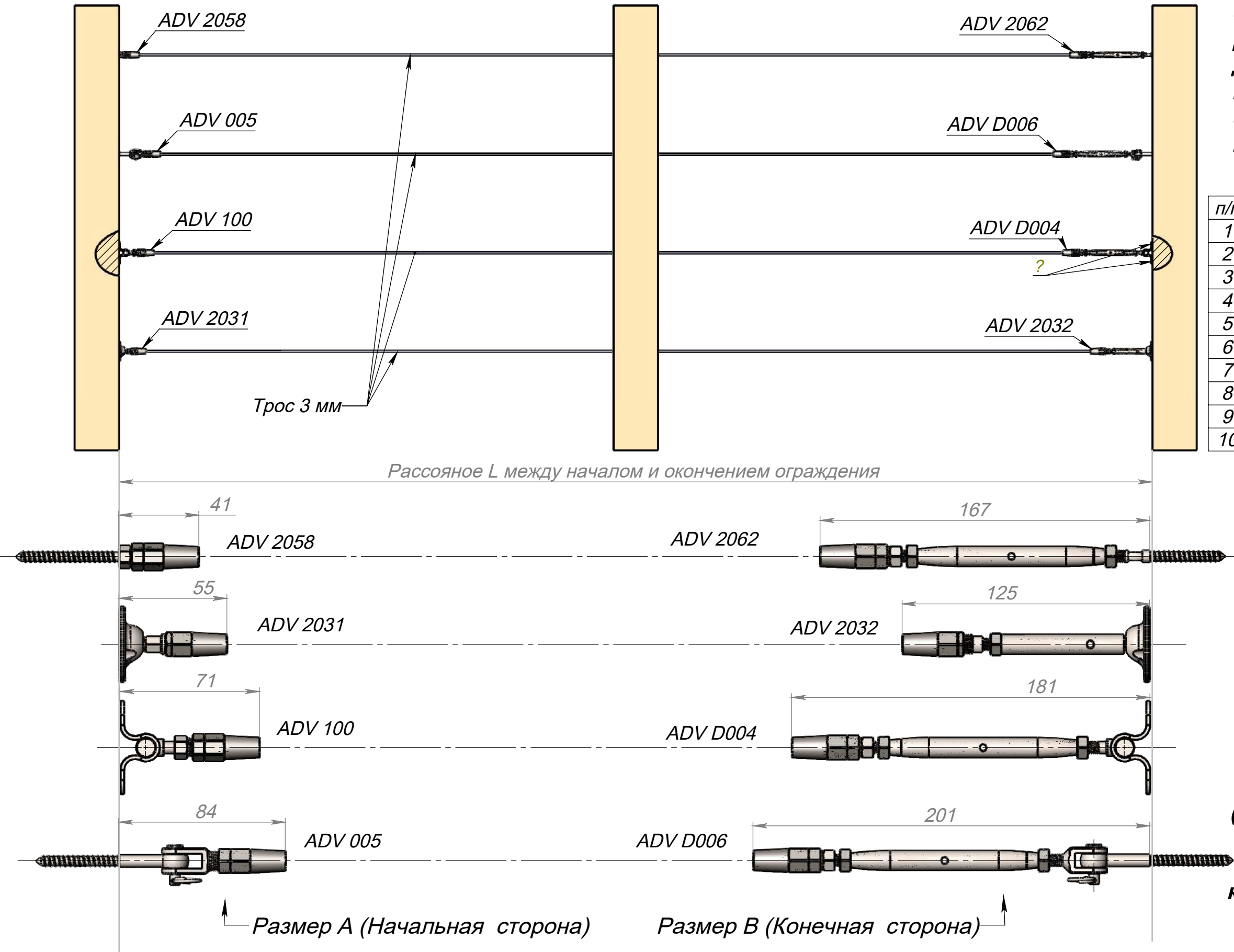
Схема 2 рекомендуемых вариантов установки системы тросов с использованием цанговых наконечников
